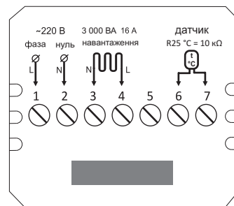
Схема 1. Схема під'єднання
