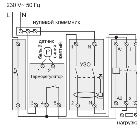
Схема 2. Подключение через контактор (магнитный пускатель)
