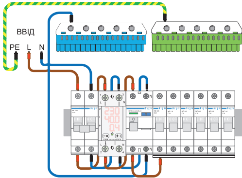
Схема 2. Варіант монтажної схеми з транзитом нуля через ZUBR MF
