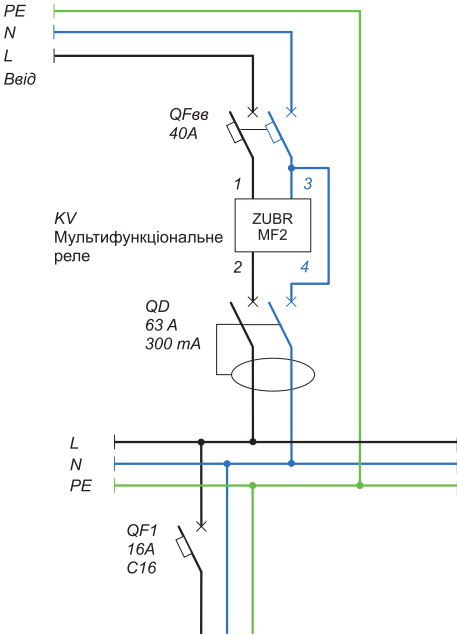
Схема 3. Варіант електричної схеми без транзитну нуля через ZUBR MF2
