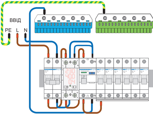
Схема 4. Варіант монтажної схеми без транзитну нуля через ZUBR MF2
