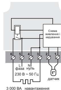
Схема 1. Схема підключення та спрощена внутрішня схема
