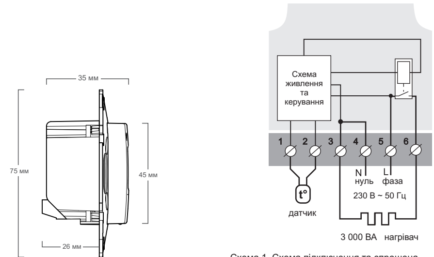
Схема 1. Схема підключення та спрощена внутрішня схема
