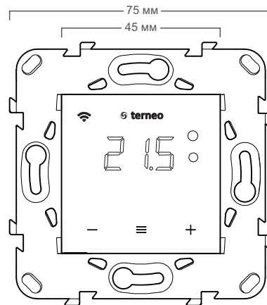
Рисунок 1. Габаритні розміри
